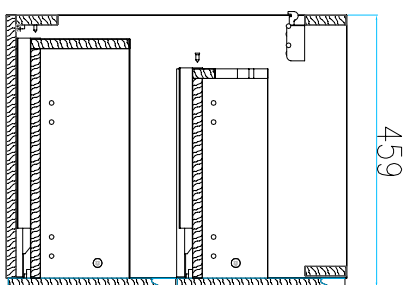
Przekrój A-A
