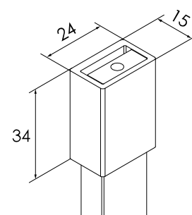
b WSPORNIK
